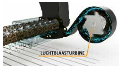
Werking van het gepatenteerde Helix Seed Duct-systeem van de Eliet DZC600 en DZC 450
